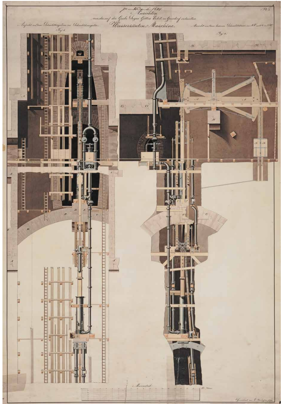
Wassersäulenmaschine der Grube Segen Gottes Erbistolln (Sächsisches Staatsarchiv, Bergarchiv Freiberg (SächsStA-F), 40044 Generalrisse, Nr. 1-K20034)
